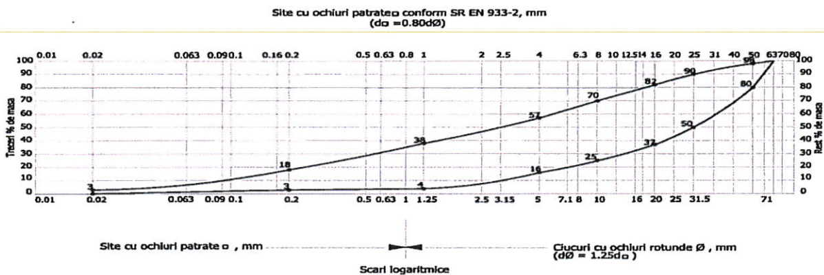
Figura 1 - Zona granulometrica prescisa pentru balastul din stratul interior de fundatie
